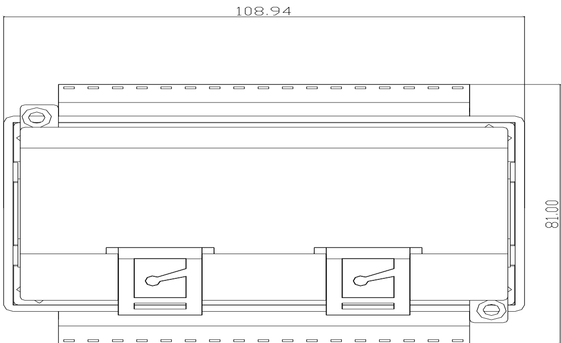
底视图
