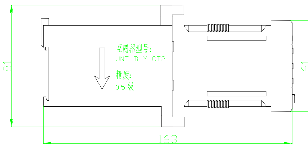
主视图
