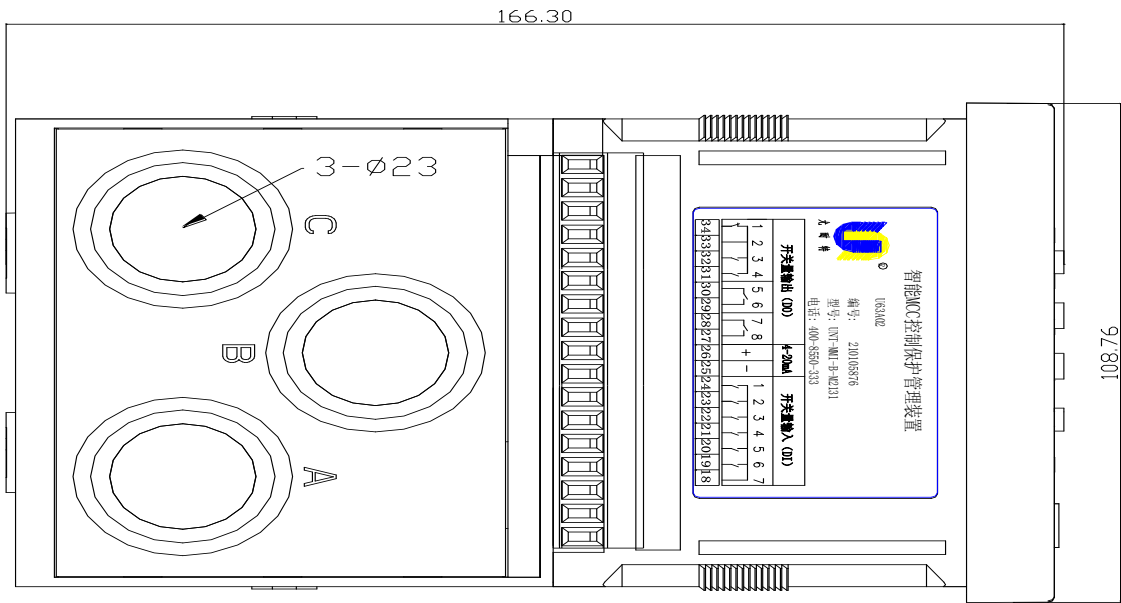
侧视图
